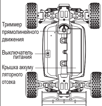
Радиоуправляемая багги
