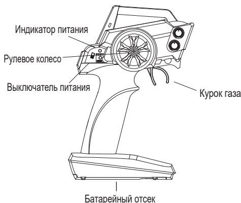
Пульт управления
